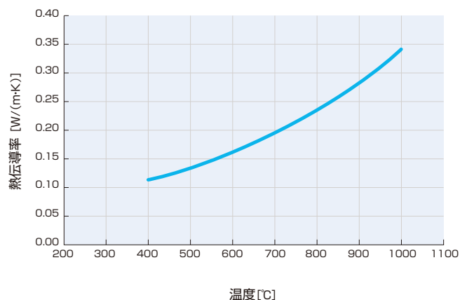
ファインフレックスBIO ブランケット (130kg/m³) の熱伝導率
